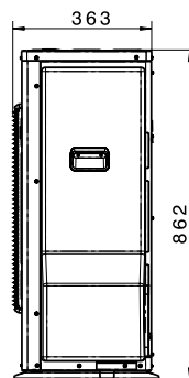
Unidad exterior BWL-1S(B)-10-14-16 vista lateral
