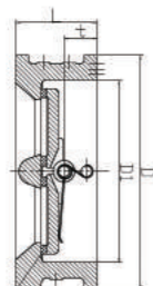
VÁLVULA RETENCIÓN TIPO RUBER CHECK PN10/16
