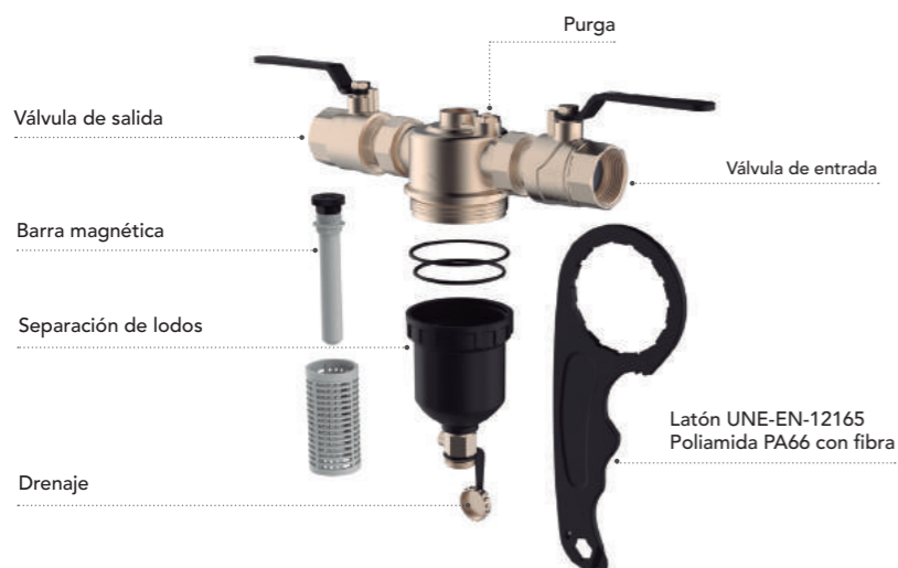
Filtro magnético de 1 ¼"
