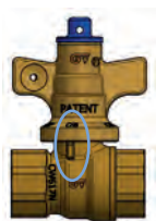
B Bloqueo en posición Abierta (OB) Lock in Open position (OB)
