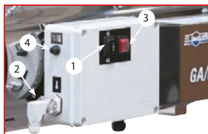
Legenda, cuadro eléctrico (IP 65) para el GA/N 45 C 1. Interruptor quemador-ventilador 2. Toma y clavija para termostato ambiente 3. Pulsador de reset (rearme) 4. Termostato de sobrecalentamiento de rearme manual
