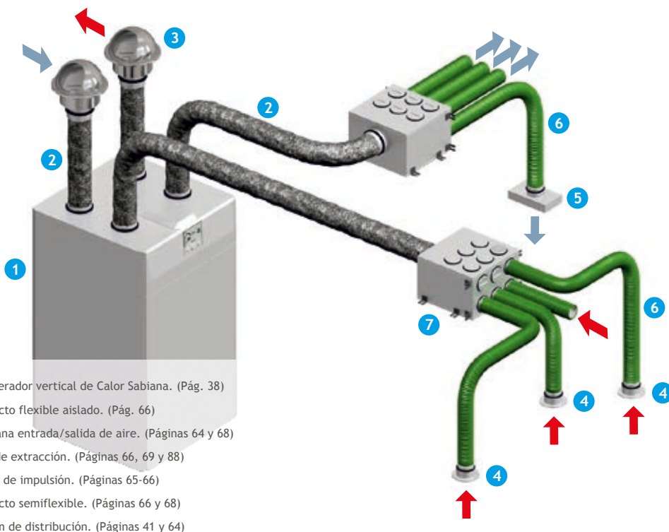
ESQUEMA TIPO VIVIENDA UNIFAMILIAR CON CONDUCTO SEMIFLEXIBLE
