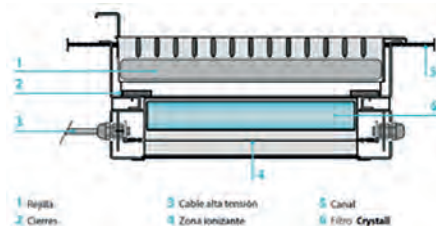
Filtro CRYSTALL difusores CDS-I
