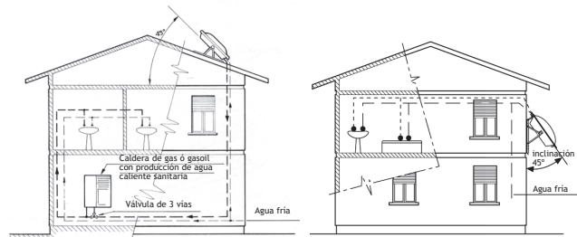
Fácil conexión a través de la caldera existente
