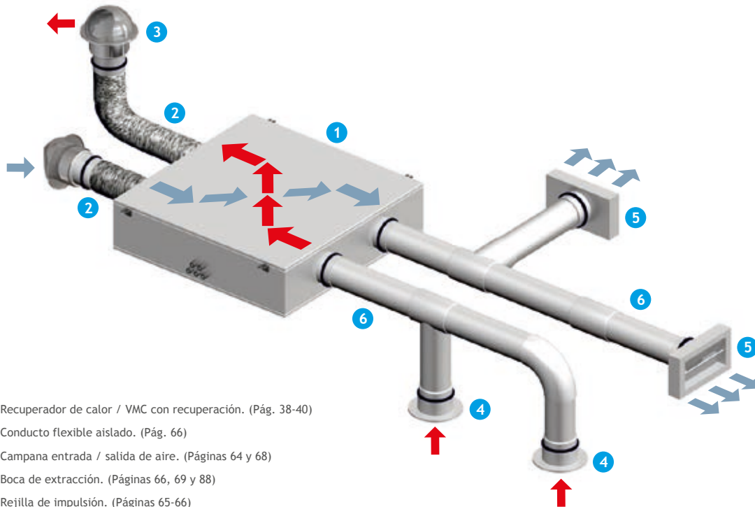
ESQUEMA TIPO VIVIENDA COLECTIVA CON CONDUCTO RÍGIDO
