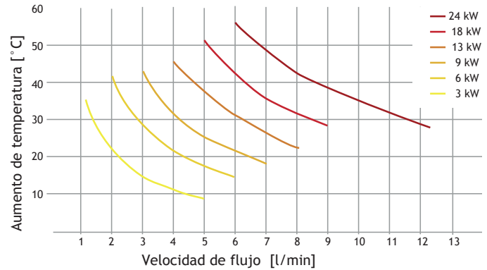
Gráfico de rendimiento instantáneo
