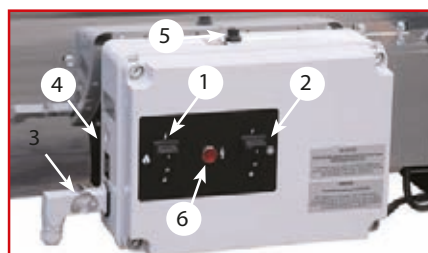
Legenda, cuadro eléctrico (IP 65) para GA/N 80 C- GA/N 100 C y GA 100 C 1. Interruptor del quemador 2. Interruptor del ventilador 3. Toma y clavija para termostato ambiente 4. Pulsador de reset con luminoso de bloqueo (rojo), funcionamiento (verde) y stand-by (naranja) 5. Termostato de sobrecalentamiento de rearme manual. 6. Luminoso de presencia de tensión. Interruptores de mando con dos posiciones: Int. 1 OFF + Int. 2 ON = solo ventilación Int. 1 ON + Int. 2 OFF = quemador encendido con post ventilación para enfriamiento de la cámara de combustión Int. 1 ON + Int. 2 ON = quemador encendido con ventilación continua.
