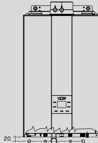
Preinstalación empotrada con plantilla Ref. 8614988 ver página 12
