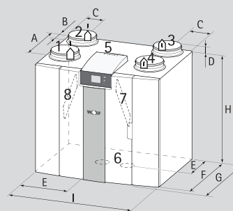
Conexiones modelo 4/0 R
