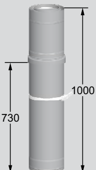
CONDUCTO CONCÉNTRICO PARA PASO DE TEJADO DN250/350
