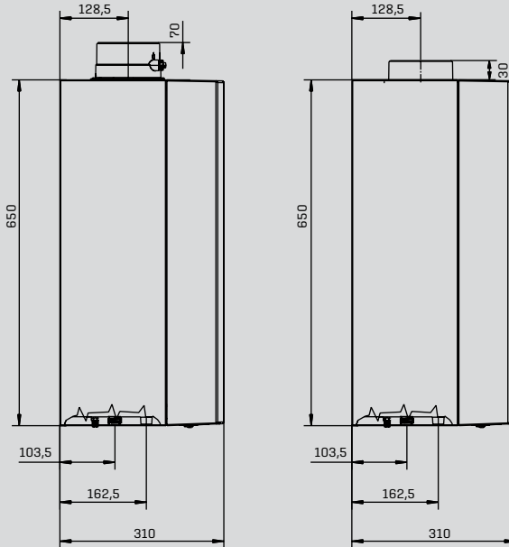
Instalación con brida de conexión 30 mm [accesorio con Ref. 173124399, ver página 18]
