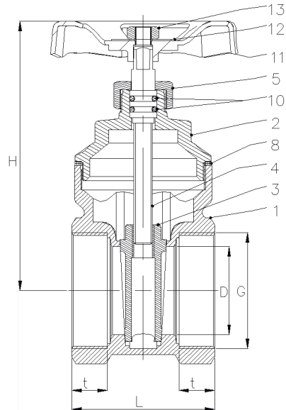
DN32 - DN100
