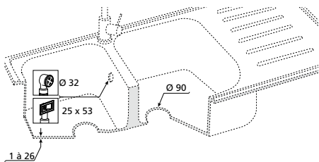
Ø 90 MM SIMPLE PARED: INOX, SINTÉTICO, CERÁMICA
